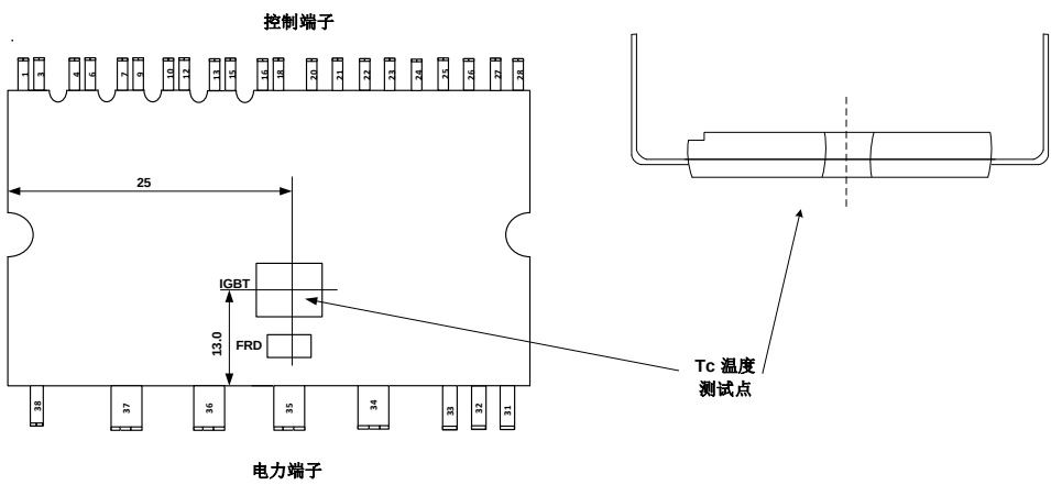
图3: 壳温测试点
