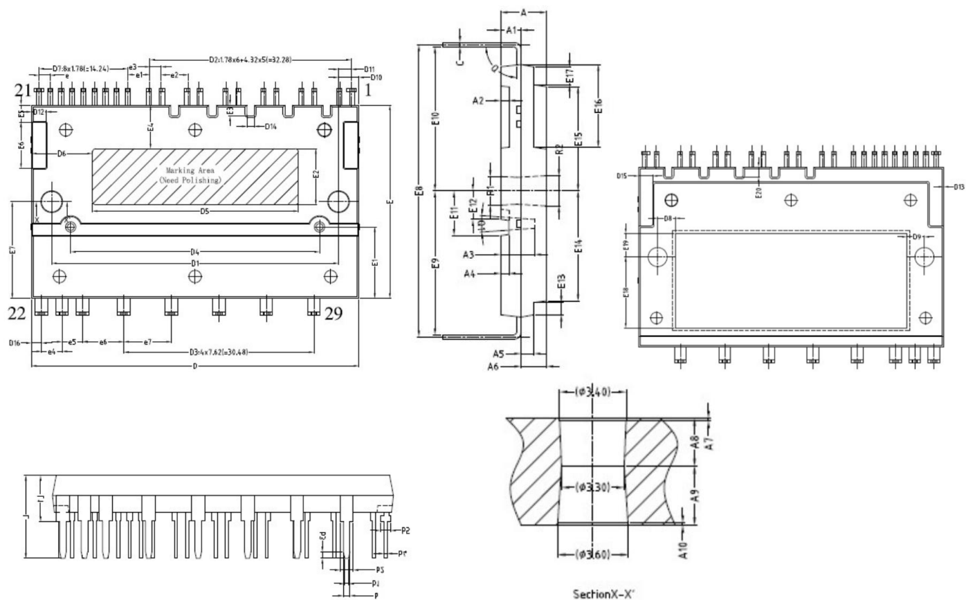
外型封装图：
