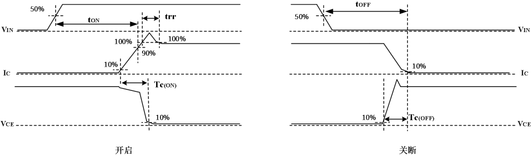
图4：开关时间定义
