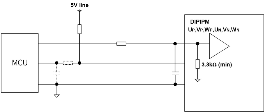
图 15：推荐的 MCU 输入输出接口电路
