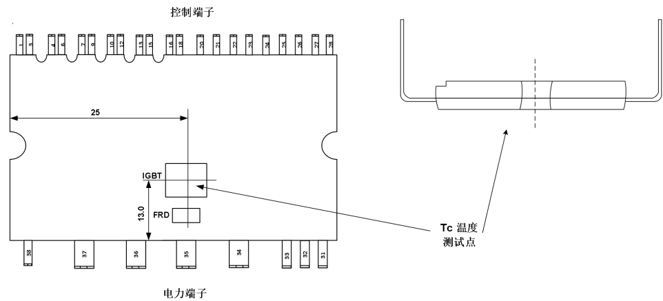
图3: 壳温测试点
