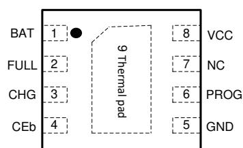
DFN3x3-8L(顶视图)
