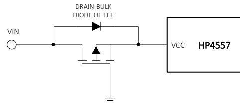
图 3：低损耗输入反向极性保护
